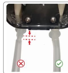
Przewód tłoczno-ssący dozowania korektora pH
